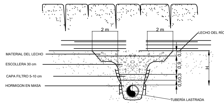
Sección A-A': Lastrado continuo
