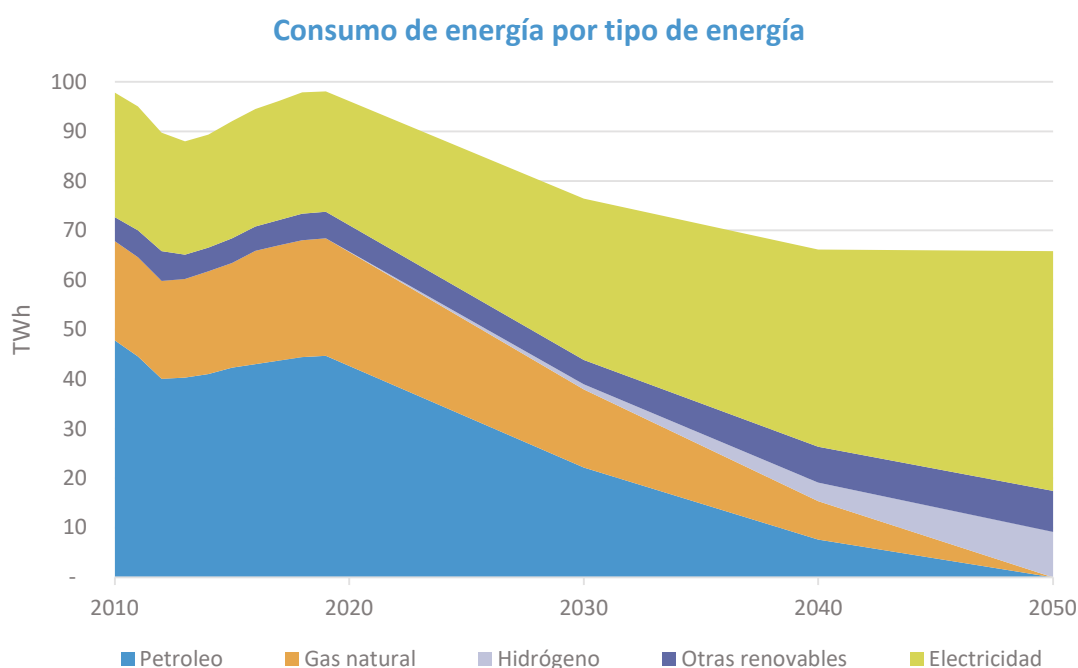
Figura 87. Prospectiva de la demanda final por tipo de energía en TWh. Fuente: elaboración propia.
