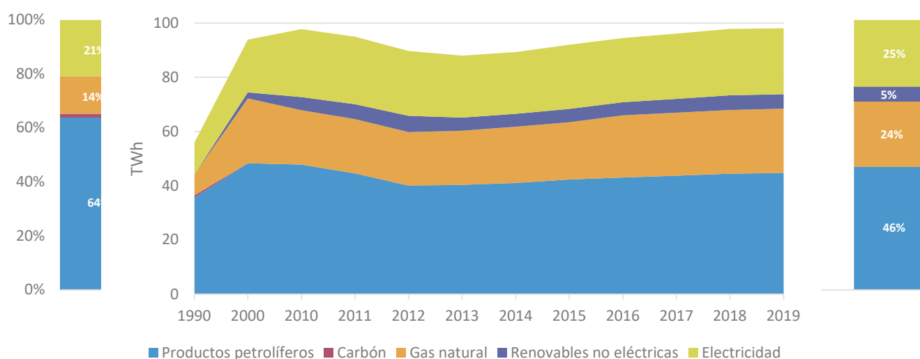
Figura 15. Evolución de la demanda de energía final en la Comunitat Valenciana en TWh. Fuente: elaboración propia con datos del IVACE.
