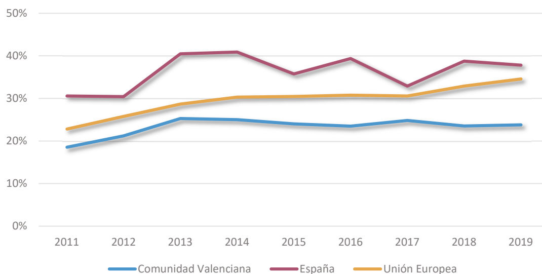
Figura 38. Evolución del porcentaje renovable en la generación de energía.
