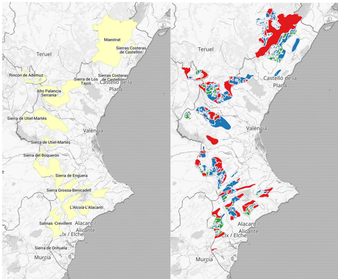
Figura 98. Áreas con potencial eólico en la Comunitat Valenciana: no aptas (rojo), condicionadas (azul) y aptas (verde). Fuente: Plan Eólico de la Comunitat Valenciana.
