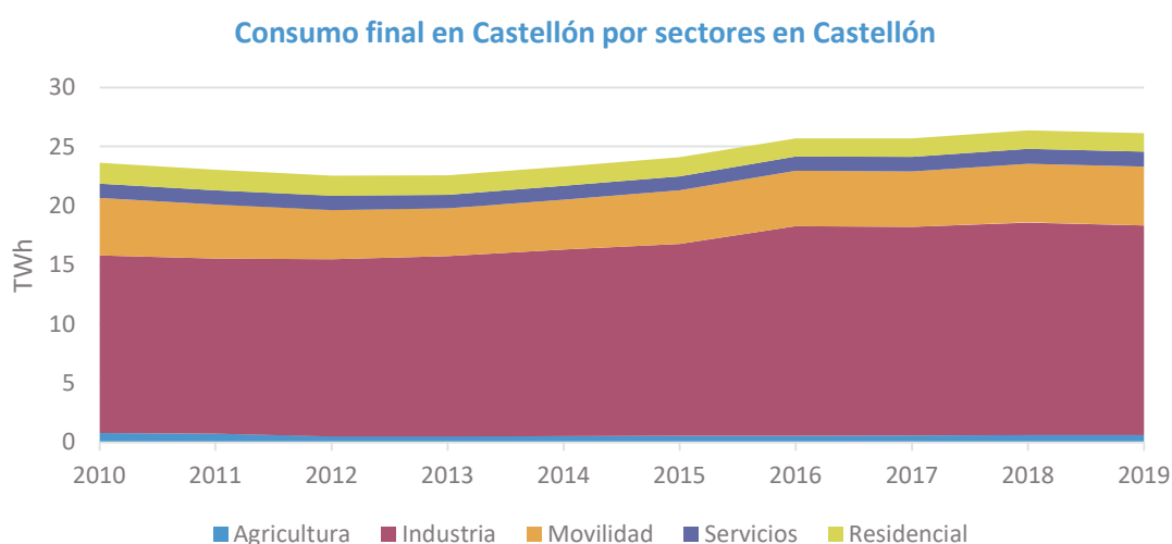
Figura 31. Evolución histórica del consumo final por sectores en Castellón.
