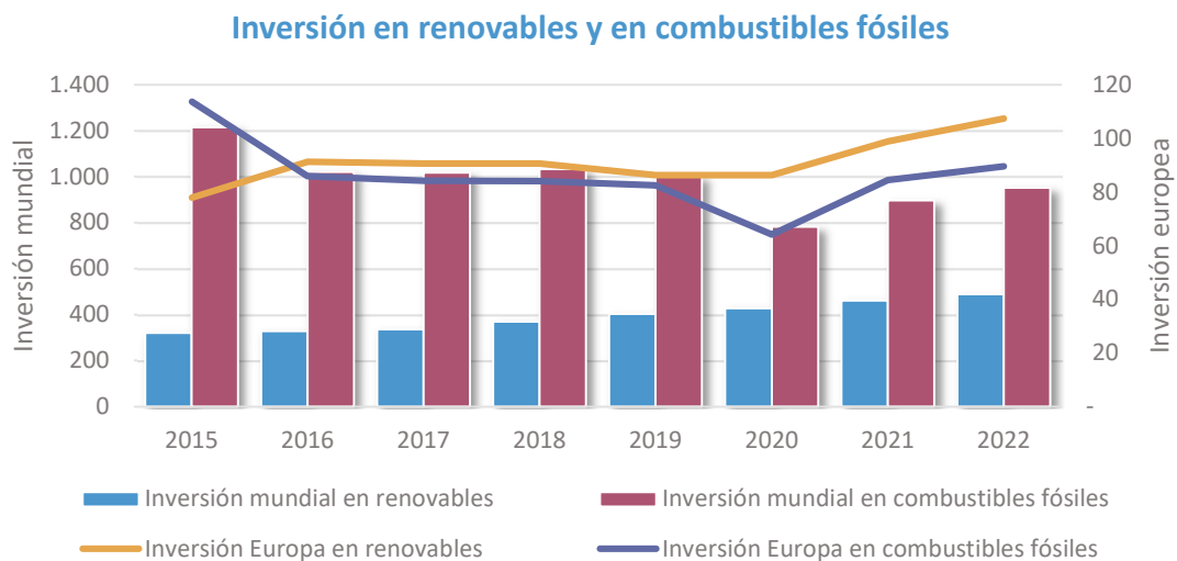
Figura 10. Variación de los diferentes flujos de inversión en renovables y en combustibles fósiles a escala mundial y europea desde 2015.
