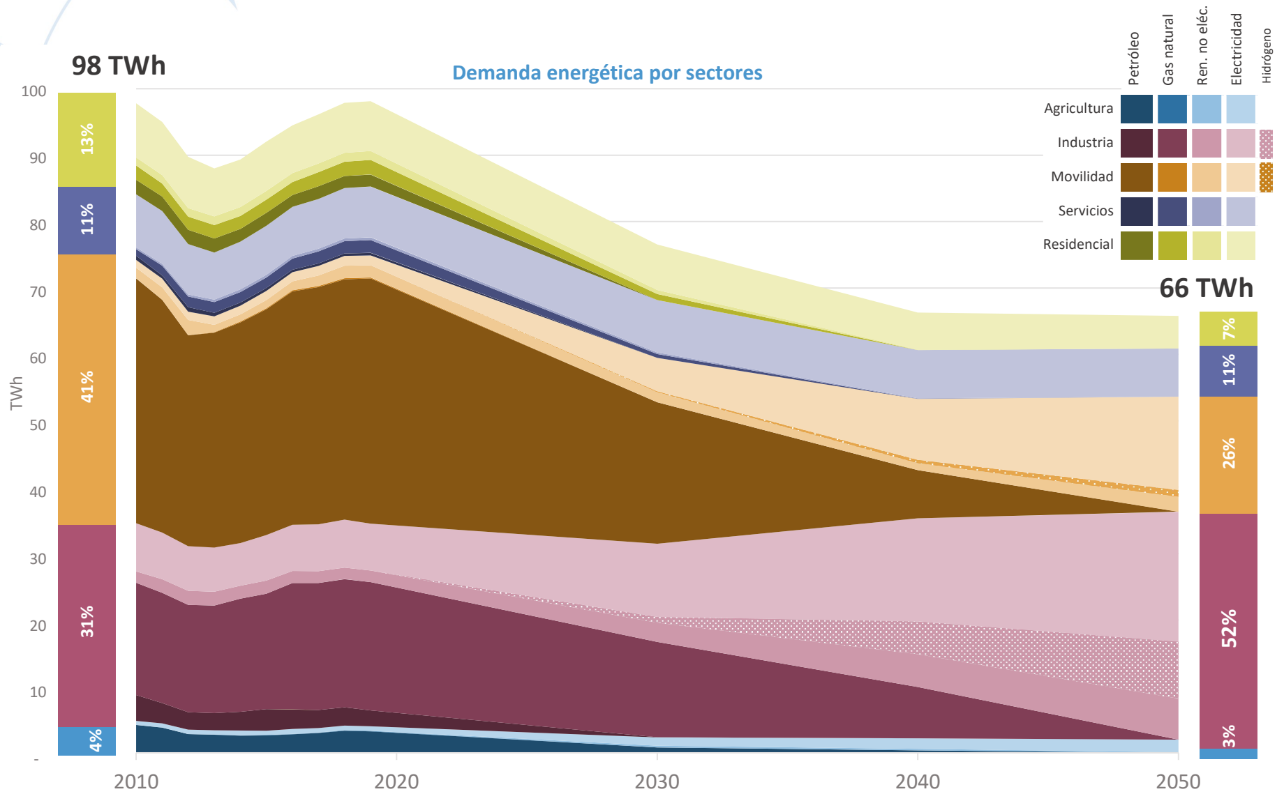
Figura 69. Demanda energética por sector y fuentes en la Comunitat Valenciana entre 2010 y 2050. Fuente: elaboración propia.
