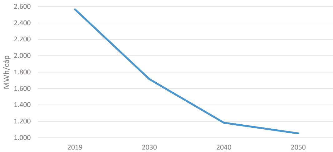
Figura 81. Prospektiva de la intensidad energética para el sector residencial. Fuente: elaboración propia.
