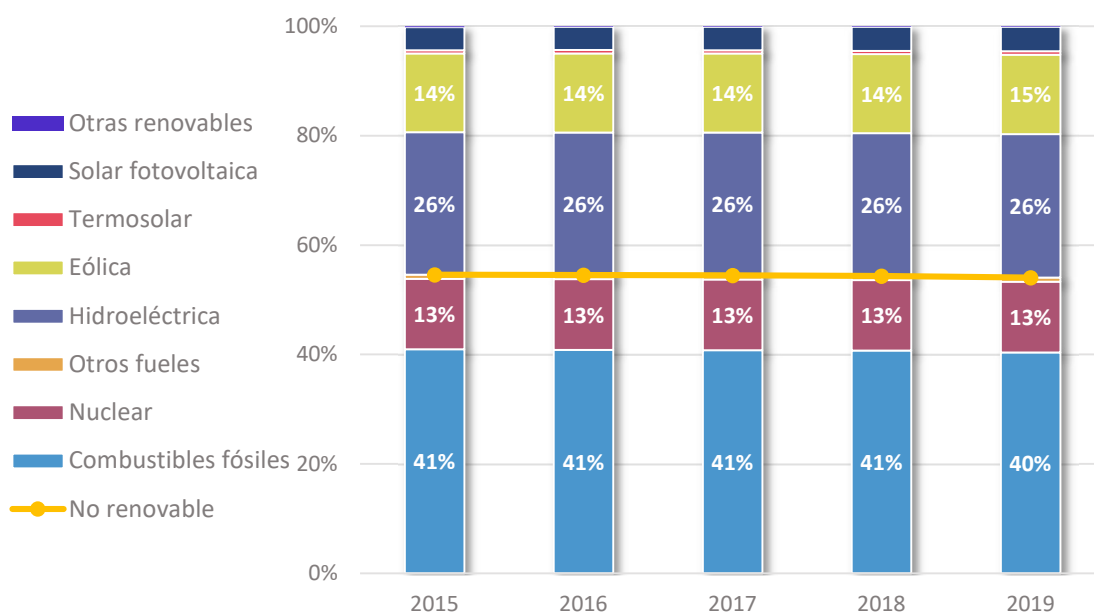
Figura 40. Evolución del porcentaje de potencia instalada por tecnología en la Comunitat Valenciana de 2015 a 2019. Fuente: elaboración propia con datos de Red Eléctrica de España.
