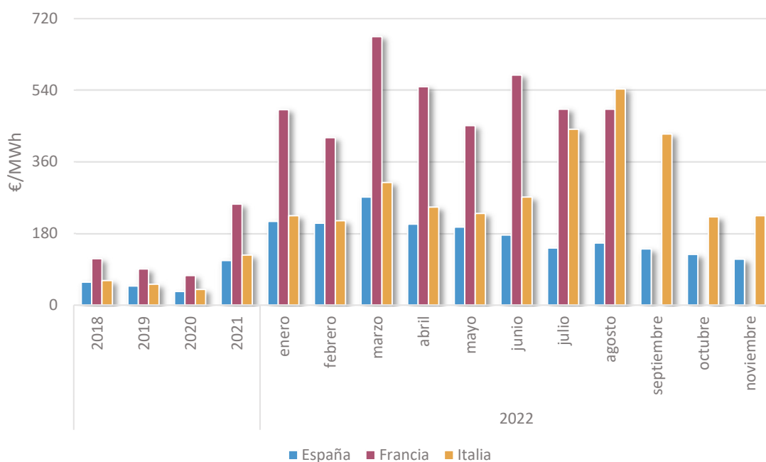
Figura 3. Precios medios (€/MWh) de los mercados mayoristas de la electricidad de España, Francia e Italia.
