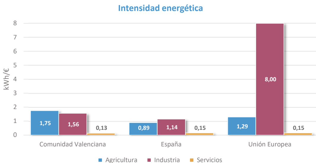
Figura 36. Comparación de intensidades energéticas en los sectores agricultura, industria y servicios en 2019. Fuente: elaboración propia con datos de Eurostat, del IVACE y del INE.
