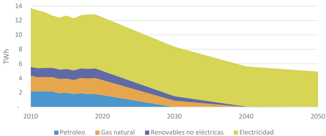
Figura 80. Prospectiva energética residencial a 2050. Fuente: elaboración propia.
