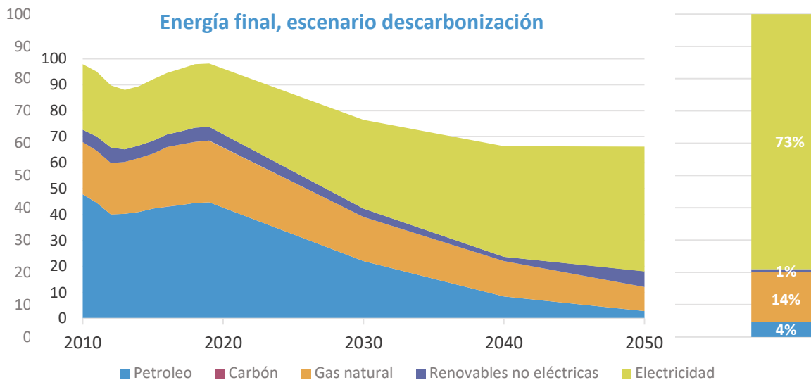
Figura 61. Pronóstico de energía final en la Comunitat Valenciana en TWh en el escenario II. Fuente: Elaboración propia.
