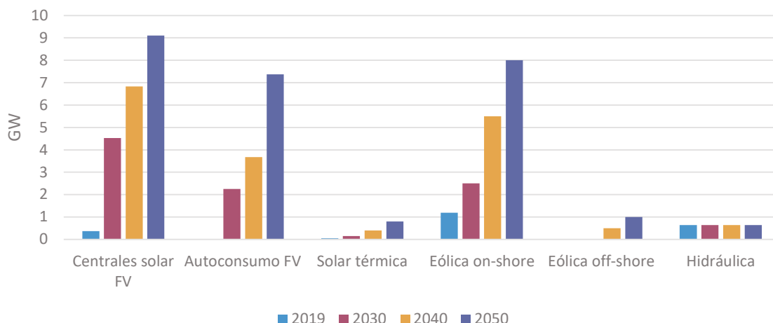
Figura 94. Potencia por tecnologías renovables. Fuente: REE y modelo Fundación Renovables.
