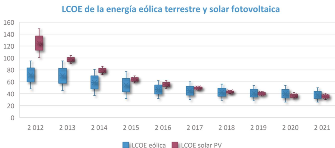
Figura 9. Evolución del LCOE de la energía eólica terrestre y solar fotovoltaica, sin subsidios, en la última década. Fuente: Lazard ( Levelized cost of energy v 15.0 ).
