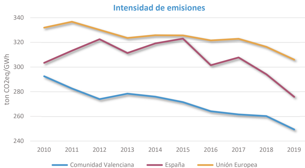
Figura 54. Intensidad de emisiones en tCO 2 eq/GWh de la Comunitat Valenciana, España y la UE entre 2010 y 2019. Fuente: elaboración propia con datos de Eurostat, del MITECO y de la Comunitat Valenciana.
