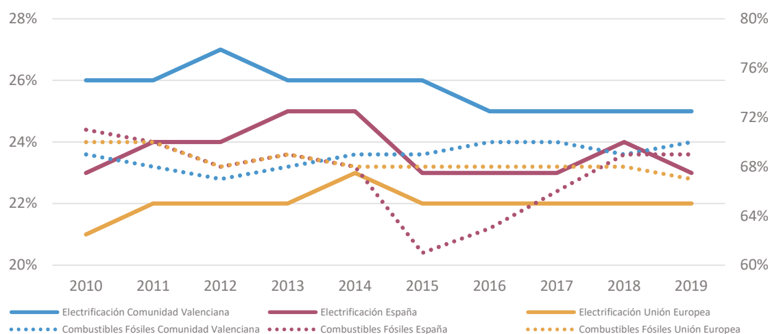
Figura 16. Grado de electrificación y porcentaje de combustibles fósiles en la Comunitat Valenciana, España y la Unión Europea. Eje izquierdo: grado de electrificación. Eje derecho: % de combustibles fósiles.
