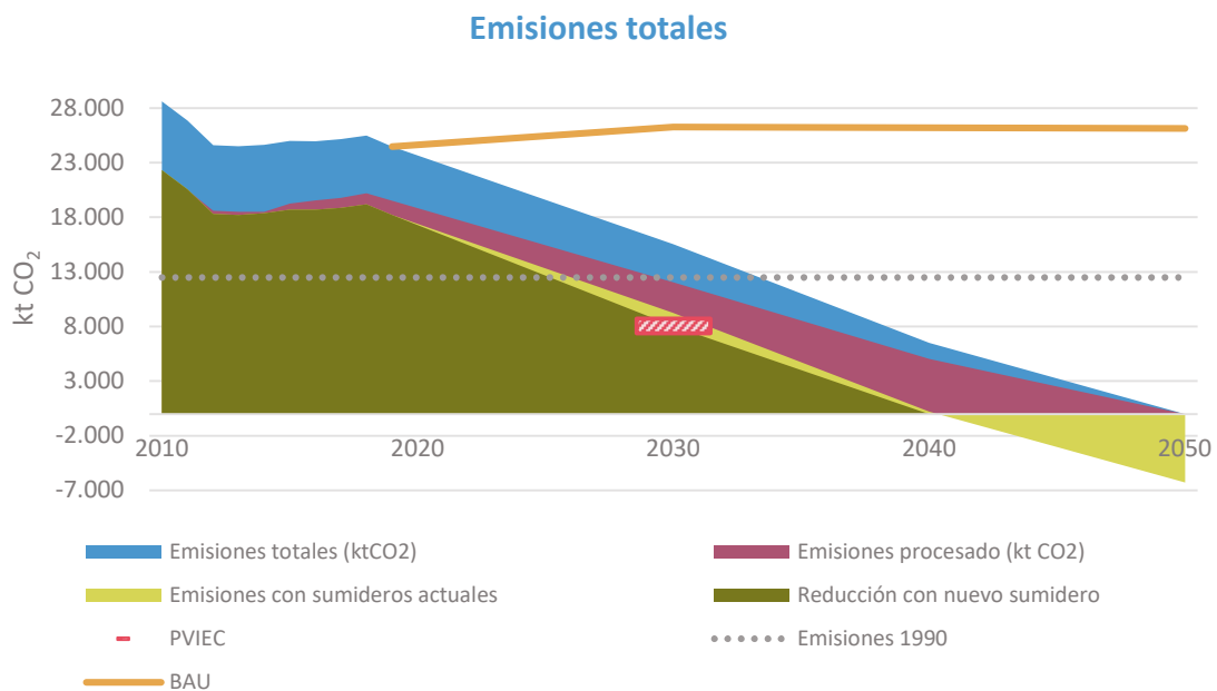
Figura 66. Pronóstico de emisiones totales y del procesado de energía en la Comunitat Valenciana en ktCO 2 eq teniendo en cuenta sumideros. Fuente: elaboración propia.
