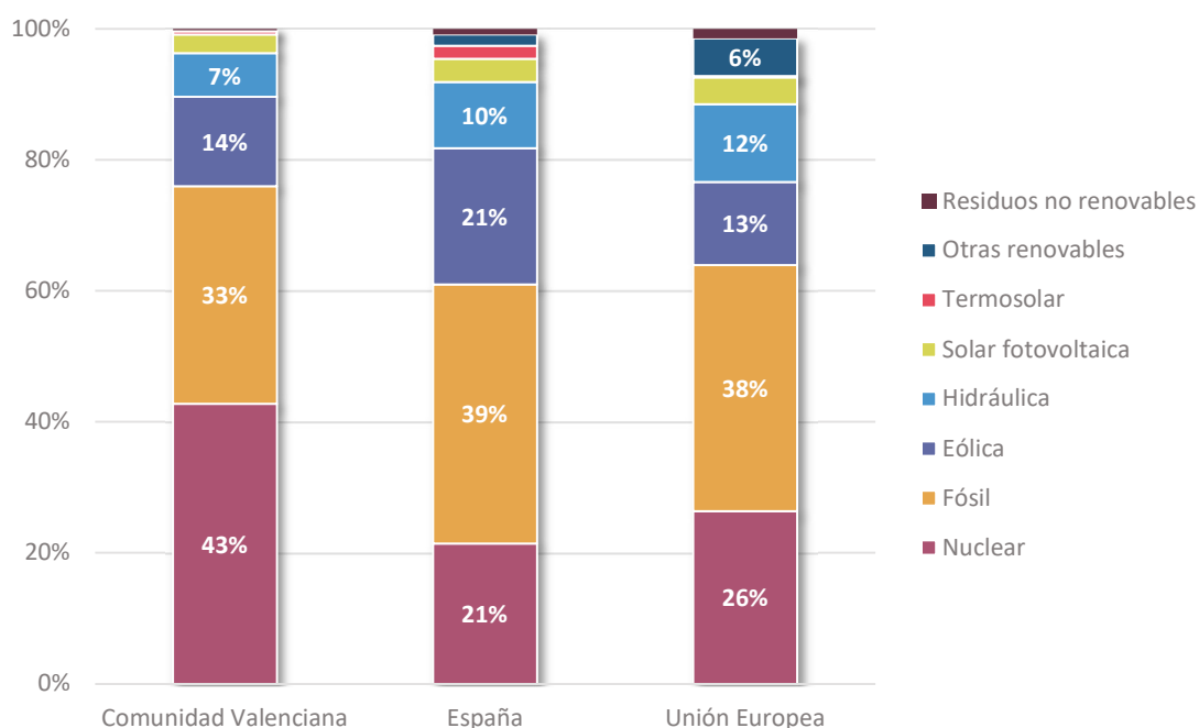
Figura 39. Comparación del mix eléctrico en la Comunitat Valenciana, España y Europa en 2019.
