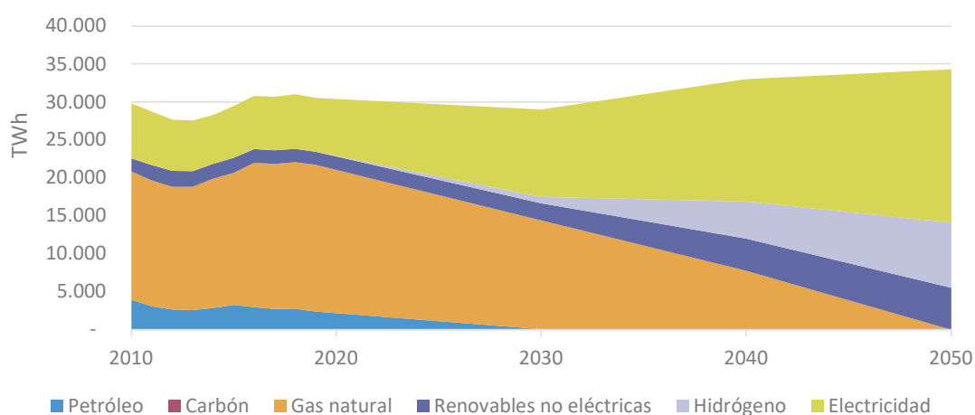
Figura 73. Prospectiva energética de la industria a 2050. Fuente: elaboración propia.
