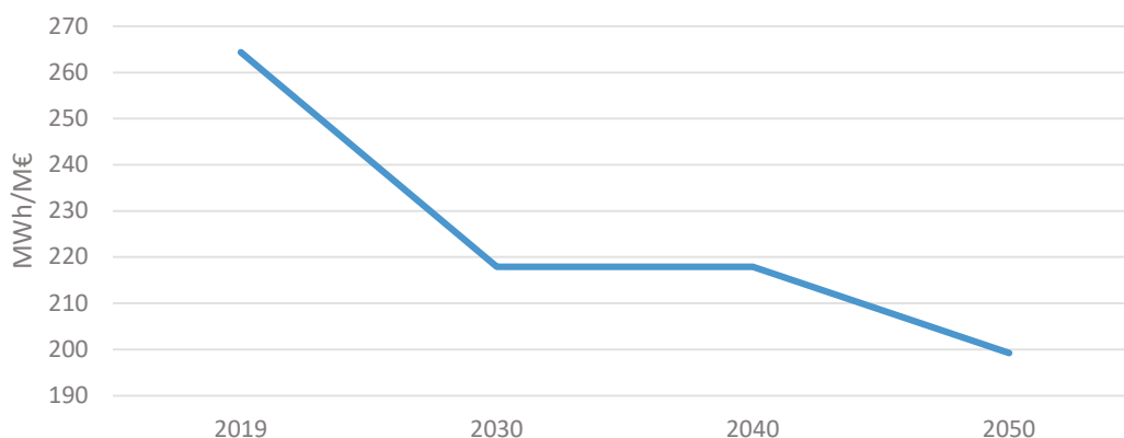
Figura 74. Prospectiva de la intensidad energética para la industria. Fuente: elaboración propia.
