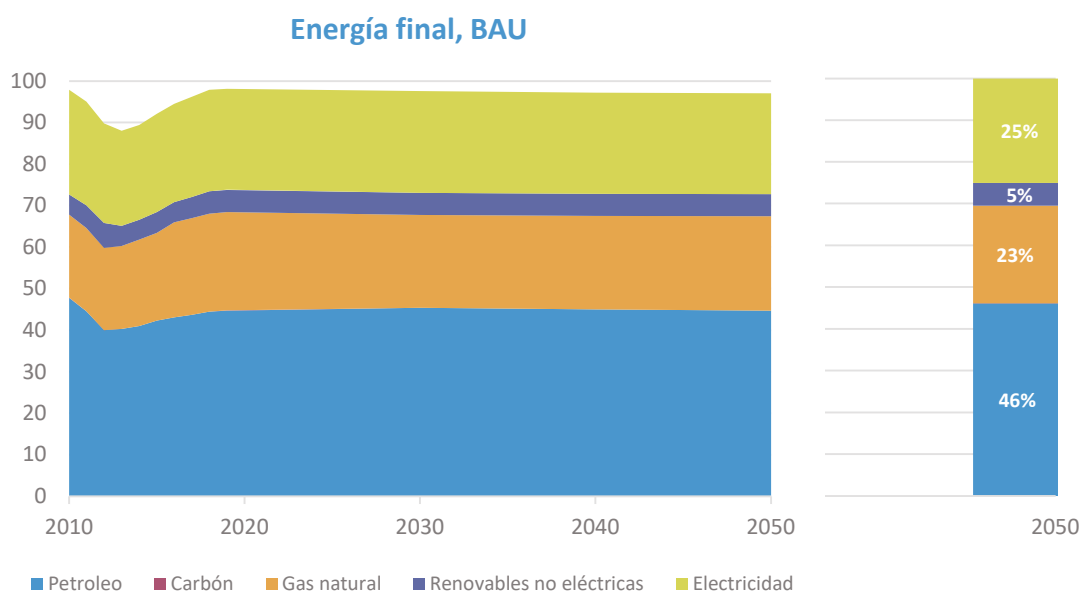
Figura 58. Pronóstico de energía final en la Comunitat Valenciana en TWh en el escenario BAU. Fuente: Elaboración propia.
