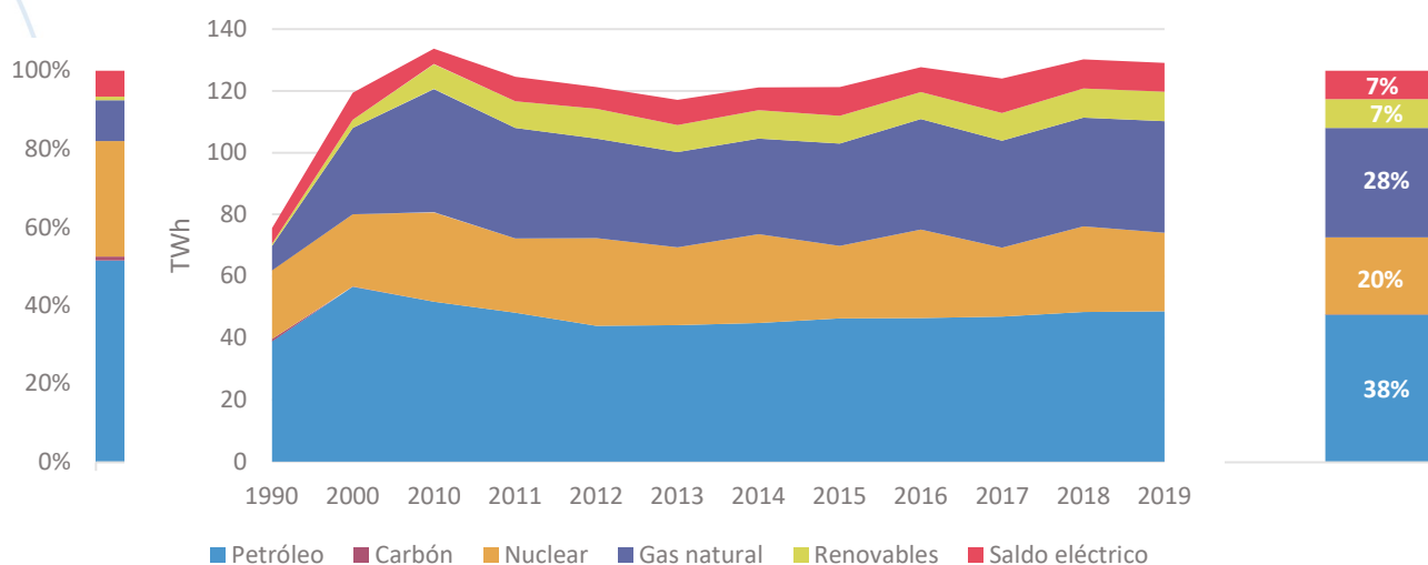
Figura 13. Evolución de la demanda de energía primaria en la Comunitat Valenciana en TWh. Fuente: elaboración propia con datos del IVACE.
