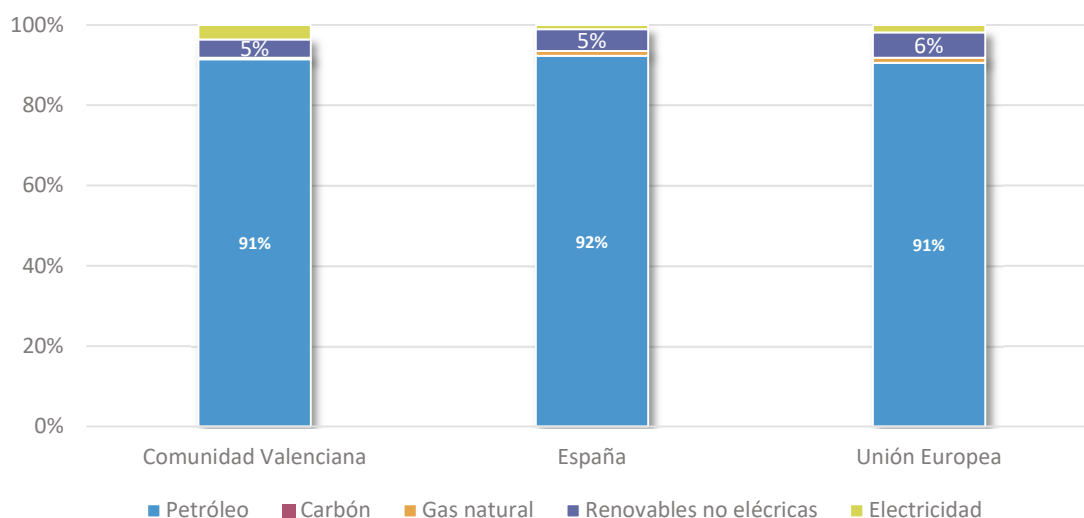
Figura 26. Comparación del consumo en transporte por fuentes en la Comunitat Valenciana en 2019.
