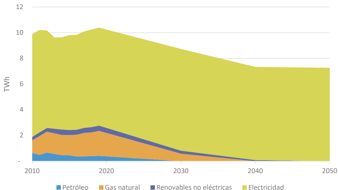
Figura 83. Prospektiva energética del sector servicios a 2050.
