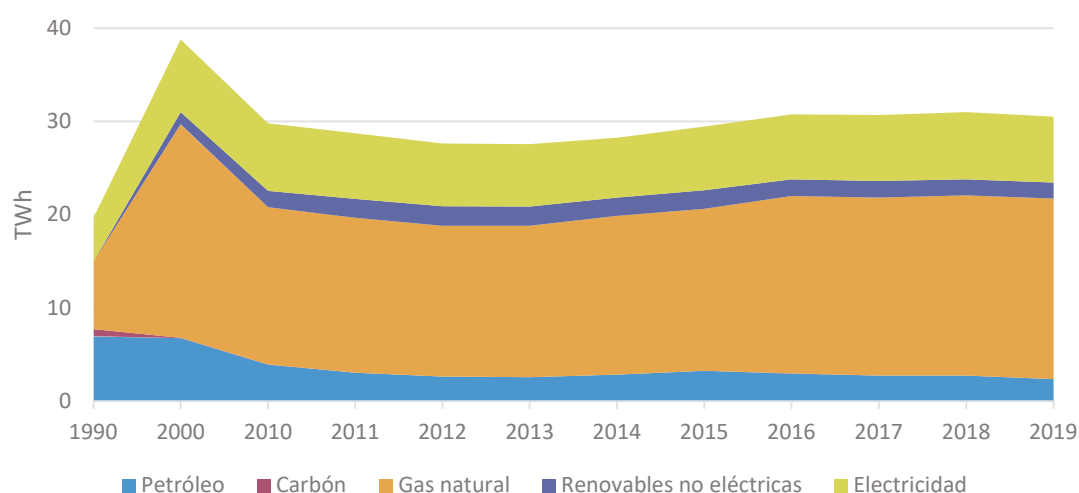
Figura 23. Evolución del consumo industrial por fuentes en la Comunitat Valenciana.
