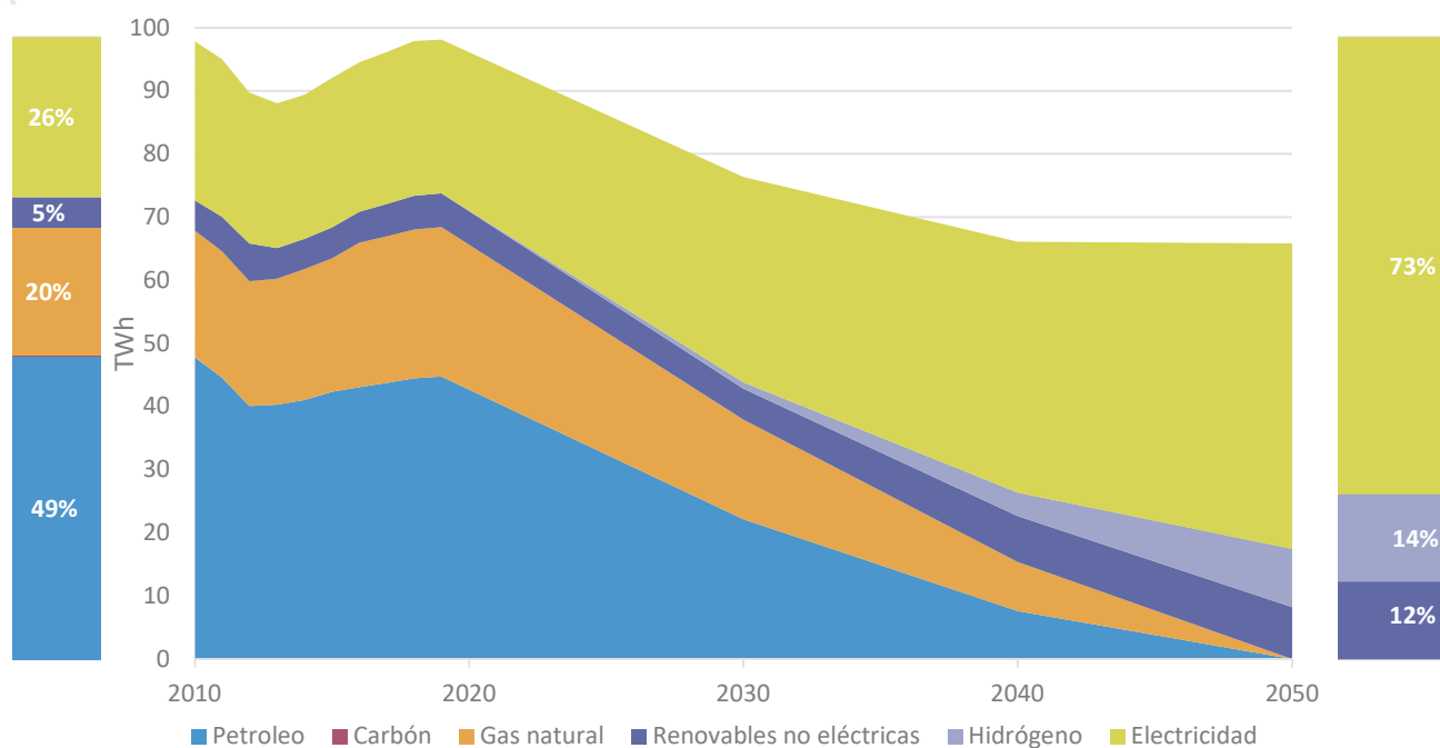
Figura 65. Pronóstico de energía final en la Comunitat Valenciana en TWh en el escenario III. Fuente: Elaboración propia.
