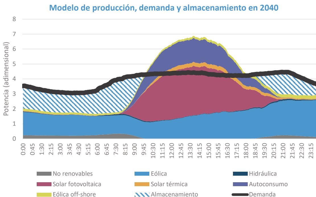
Figura 95. Representación gráfica horaria de las curvas de demanda y producción por tecnologías en un día medio para el año 2040.
