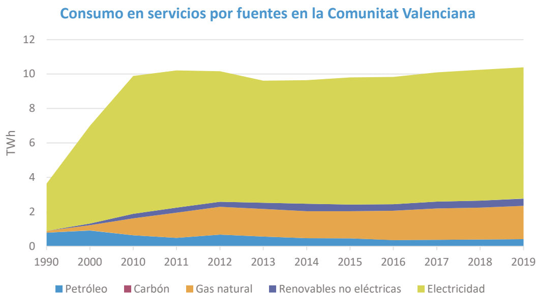
Figura 27. Evolución del consumo en servicios por fuentes en la Comunitat Valenciana. Fuente: elaboración propia con datos del IVACE.
