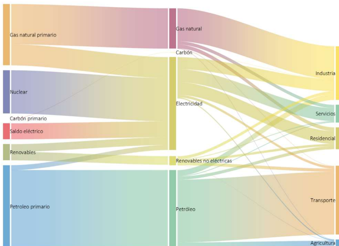
Figura 17. Diagrama de Sankey de fuentes primarias en la Comunitat Valenciana en 2019.
