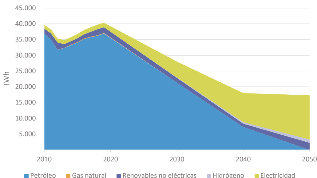
Figura 77. Prospectiva energética del transporte a 2050. Fuente: elaboración propia.
