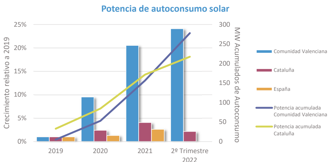
Figura 46. En barras, el crecimiento de potencia de autoconsumo solar respecto a 2019 y en líneas el número acumulado de instalaciones fotovoltaicas de La Comunitat Valenciana, Cataluña y España. Barras – eje izquierdo. Líneas – eje derecho.
