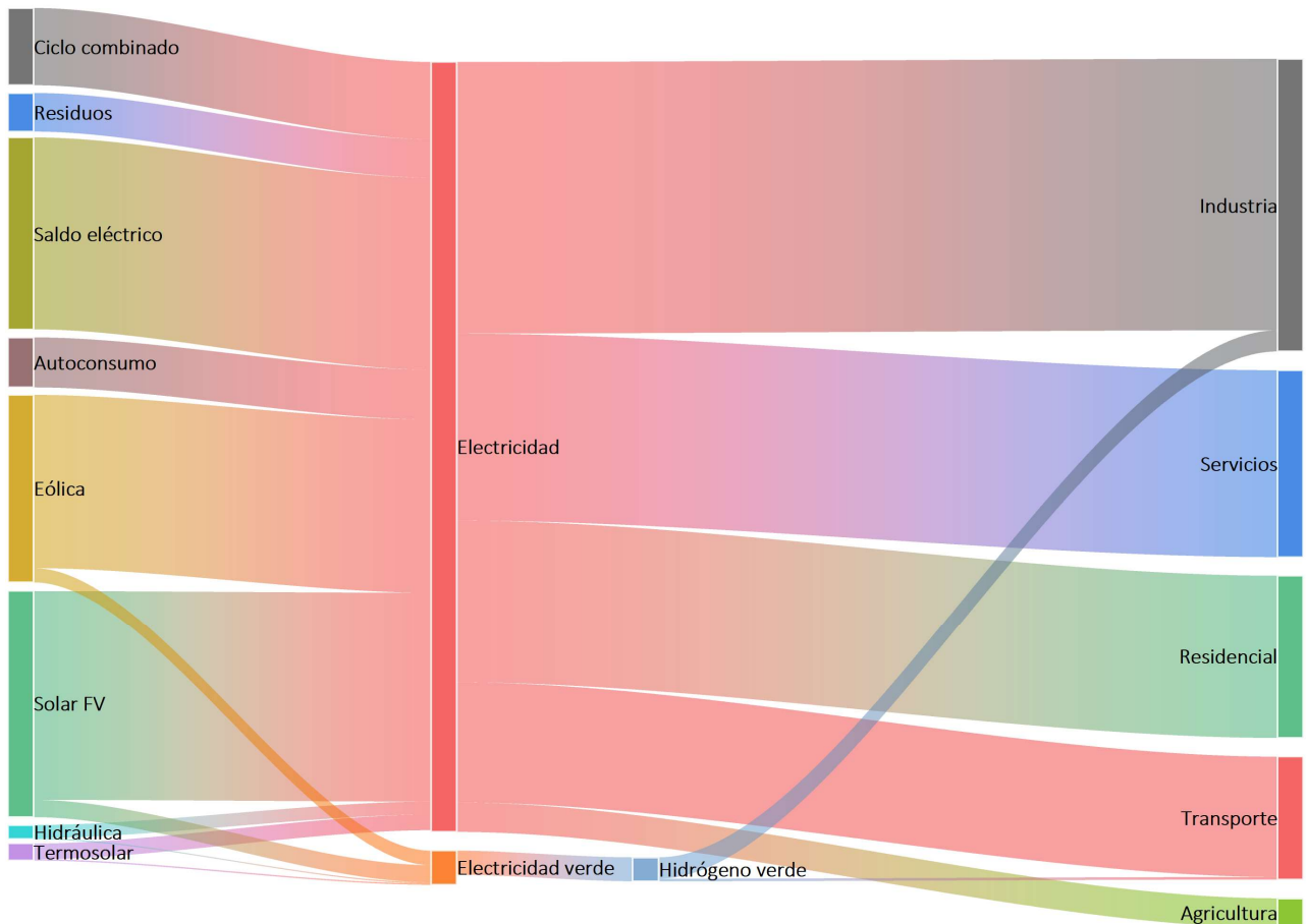
Figura 91. Fuentes, transformaciones y usos de la electricidad en la prospectiva del año 2030. Fuente: Modelo Fundación Renovables. Elaboración propia. 22
