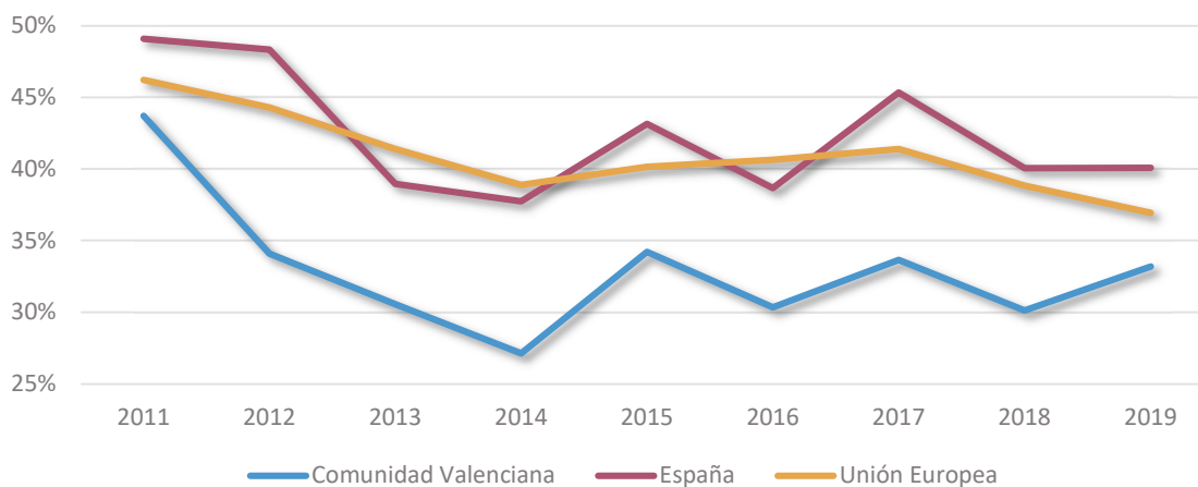
Figura 43. Evolución del % de fuentes fósiles en la potencia de generación eléctrica. Fuente: elaboración propia con datos de Red Eléctrica de España.
