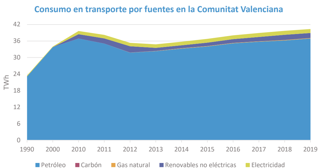
Figura 25. Evolución del consumo por fuentes en transporte en la Comunitat Valenciana.
