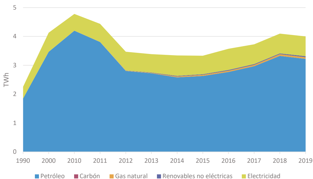
Figura 21. Evolución del consumo en agricultura por fuentes en la Comunitat Valenciana. Fuente: elaboración propia con datos del IVACE.
