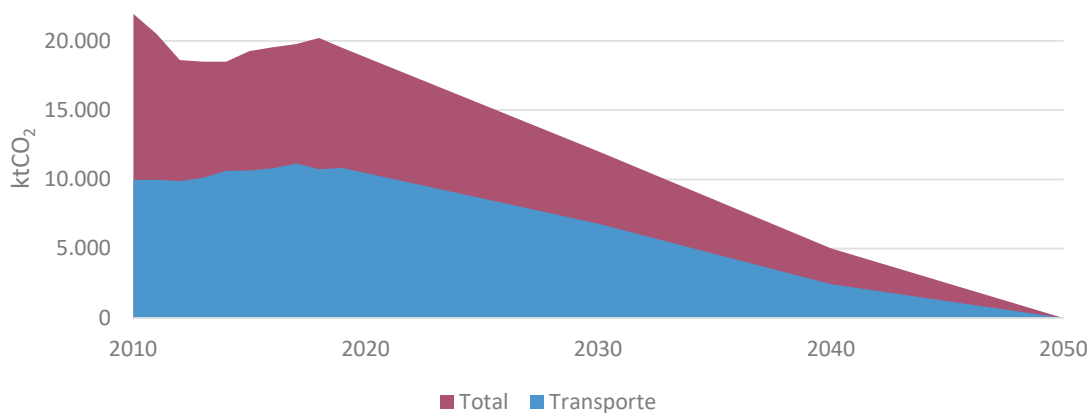
Figura 79. Prospektiva de las emisiones para el transporte. Fuente: elaboración propia.
