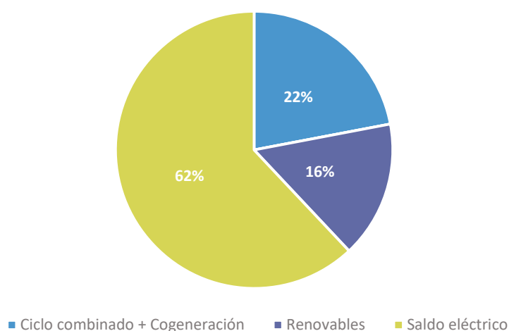
Figura 59. Mix eléctrico en el 2050 en escenario BAU. Fuente: elaboración propia. Fuente: Elaboración propia.
