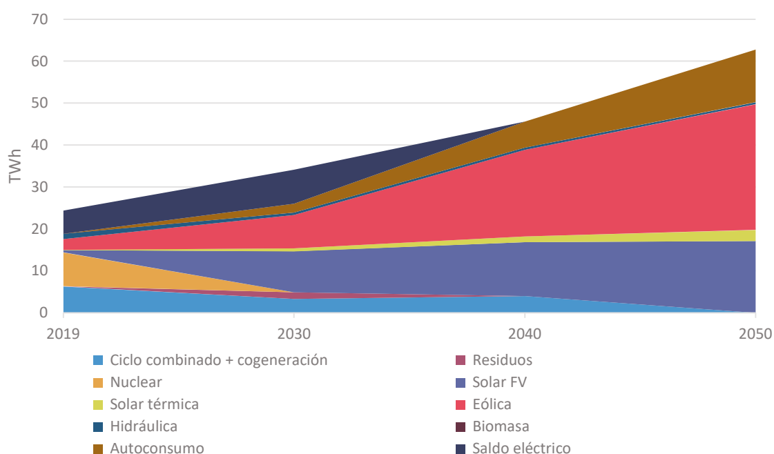
Figura 93. Prospectiva de producción de electricidad por tecnologías. Fuente: elaboración propia.
