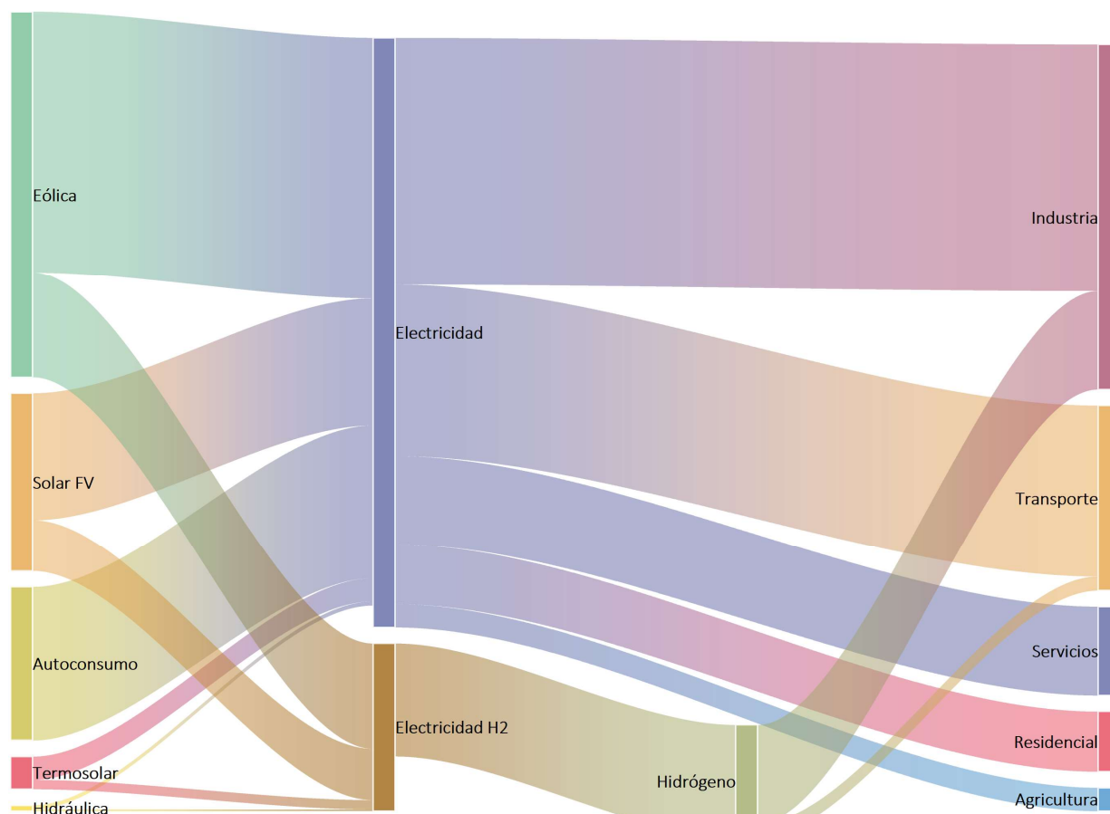
Figura 92. Fuentes, transformaciones y usos de la electricidad en la prospectiva del año 2050. Fuente: Modelo Fundación Renovables. Elaboración propia. 23
