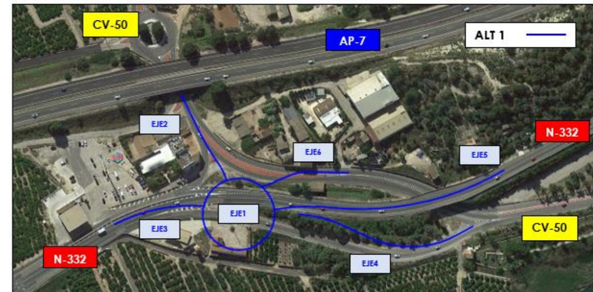
Imagen 28. Planta sobre ortofoto de la alternativa 1 de conexión con la N-332.
