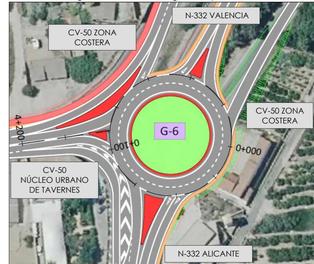
Imagen 15. Ubicación de la glorieta 6 y sus ramales.
