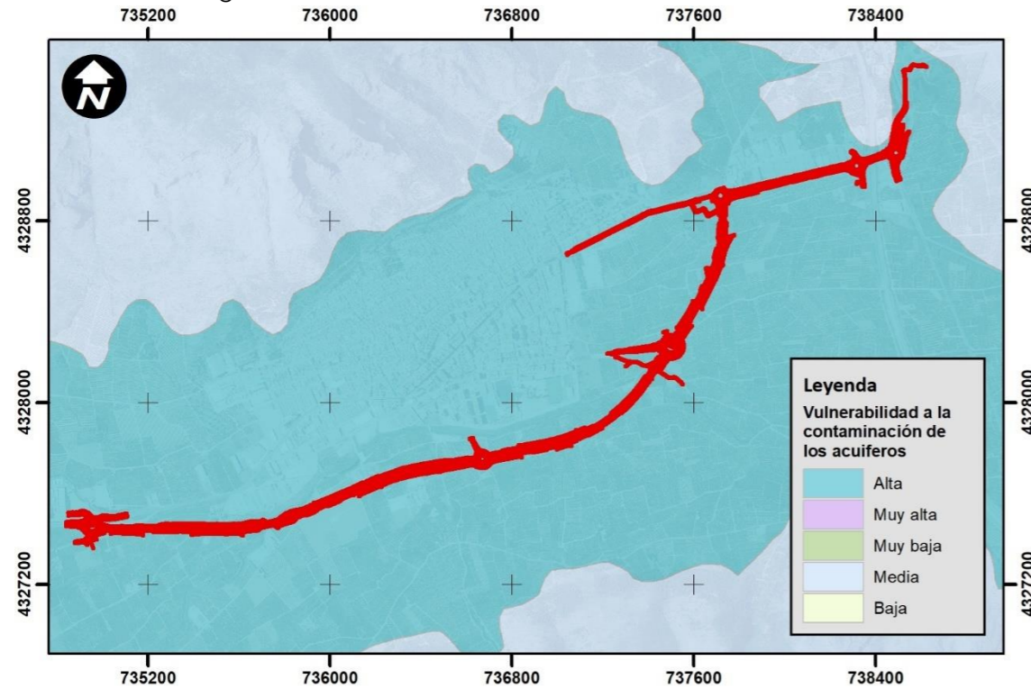
Imagen 39. Vulnerabilidad a la contaminación de acuíferos.
