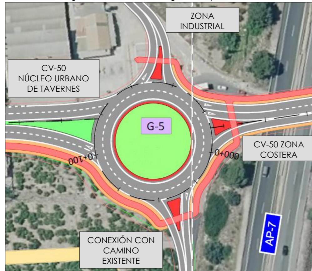
Imagen 14. Ubicación de la glorieta 5 y sus ramales.
