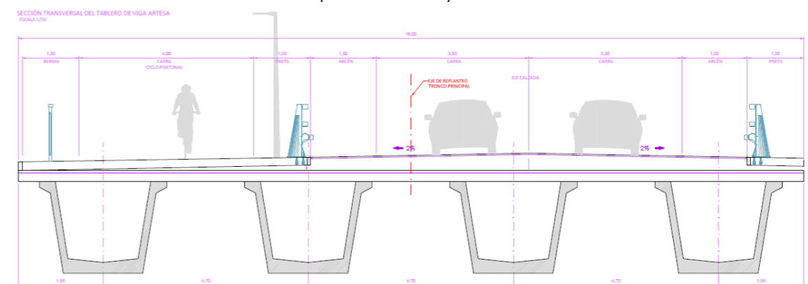
Imagen 17. Sección tipo del tablero de vigas en artesa prefabricadas para los pasos superiores EST-8 y EST-23.
