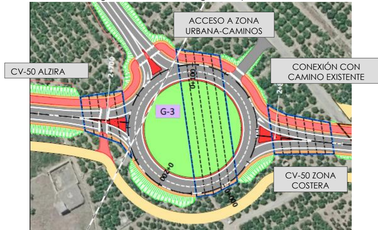
Imagen 12. Ubicación de la glorieta 3 y sus ramales.
