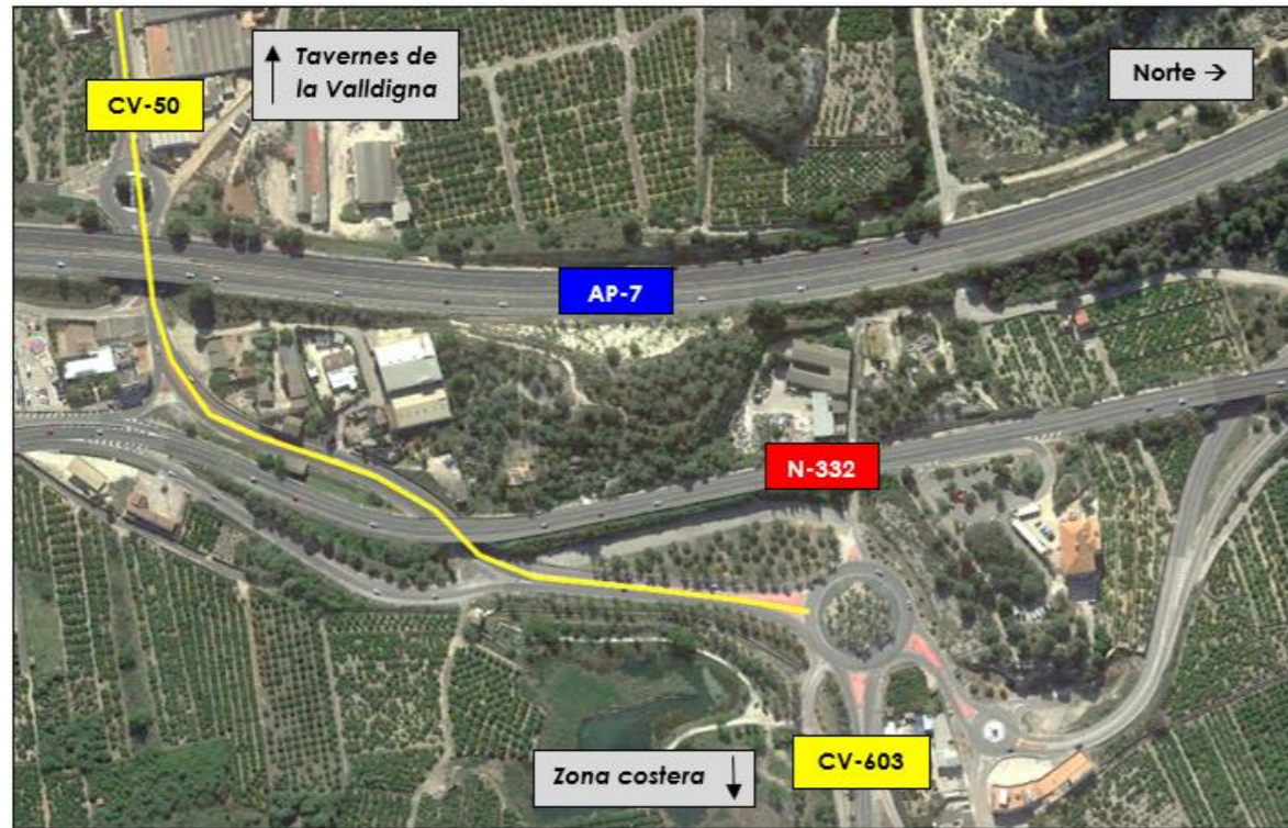
Imagen 23. Planta sobre ortofoto de la conexión actual con la N-332.
