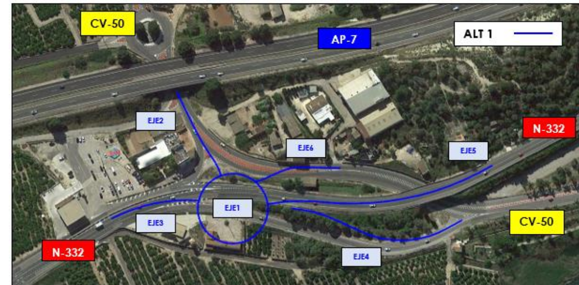
Imagen 66. Planta sobre ortofoto de la alternativa 1 de conexión con la N-332.
