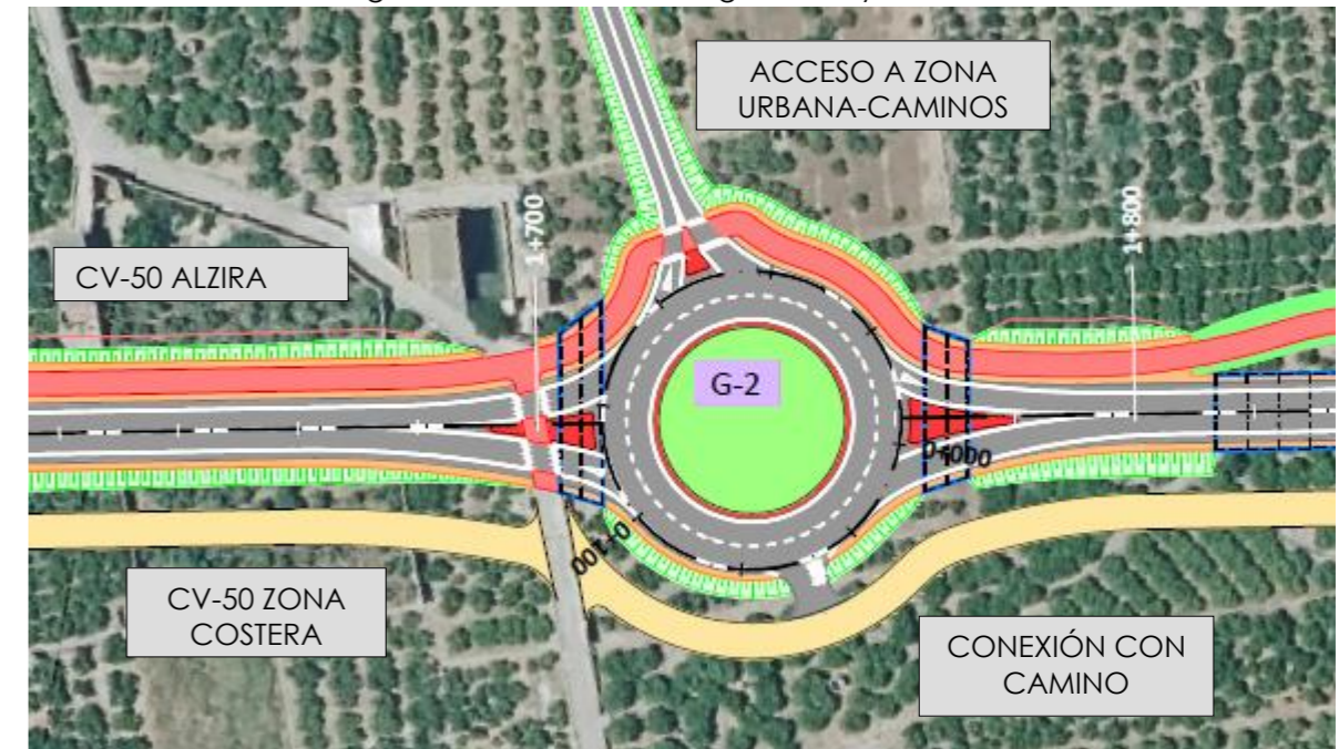
Imagen 11. Ubicación de la glorieta 2 y sus ramales.
