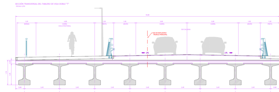
Imagen 16. Sección tipo del tablero de vigas pretensadas doble "T" para los pasos superiores est-5, est-24 y est-34.
