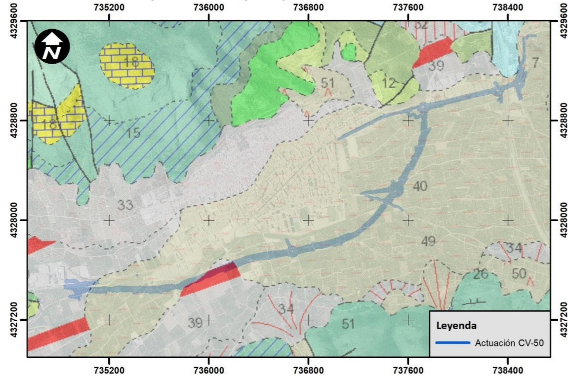
Imagen 33. Mapa geológico del ámbito de actuación.
