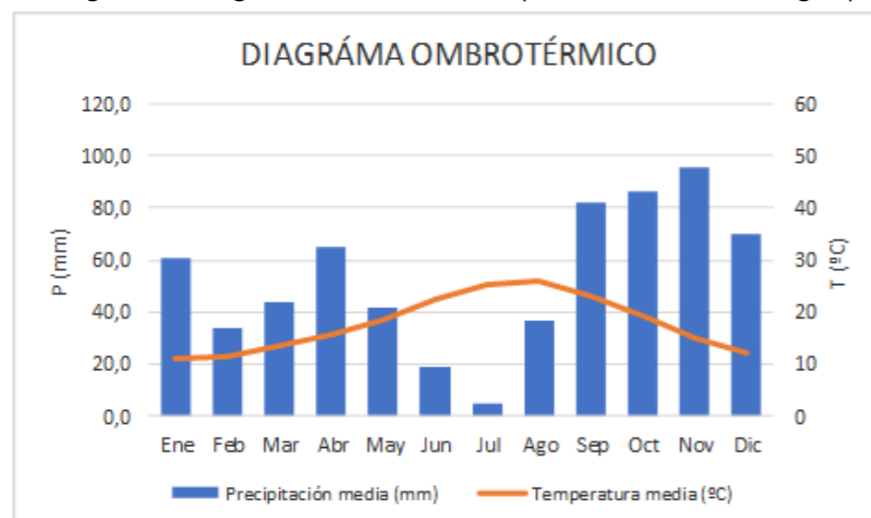
Imagen 31. Diagrama ombrotérmico (Tavernes de la Vallidigna).
