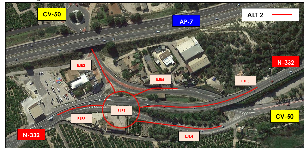
Imagen 67. Planta sobre ortofoto de la Alternativa 2 de conexión con la N-332.
