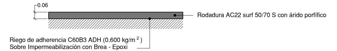
DETALLE 4 - FIRME sobre tableros de estructuras.
