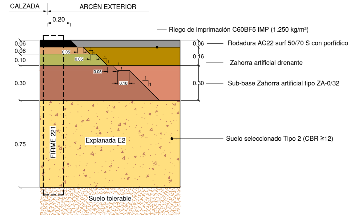
DETALLE 2 – FIRME 2221: Arcenes ejes 1, 2, y 3 y exteriores de glorietas.
