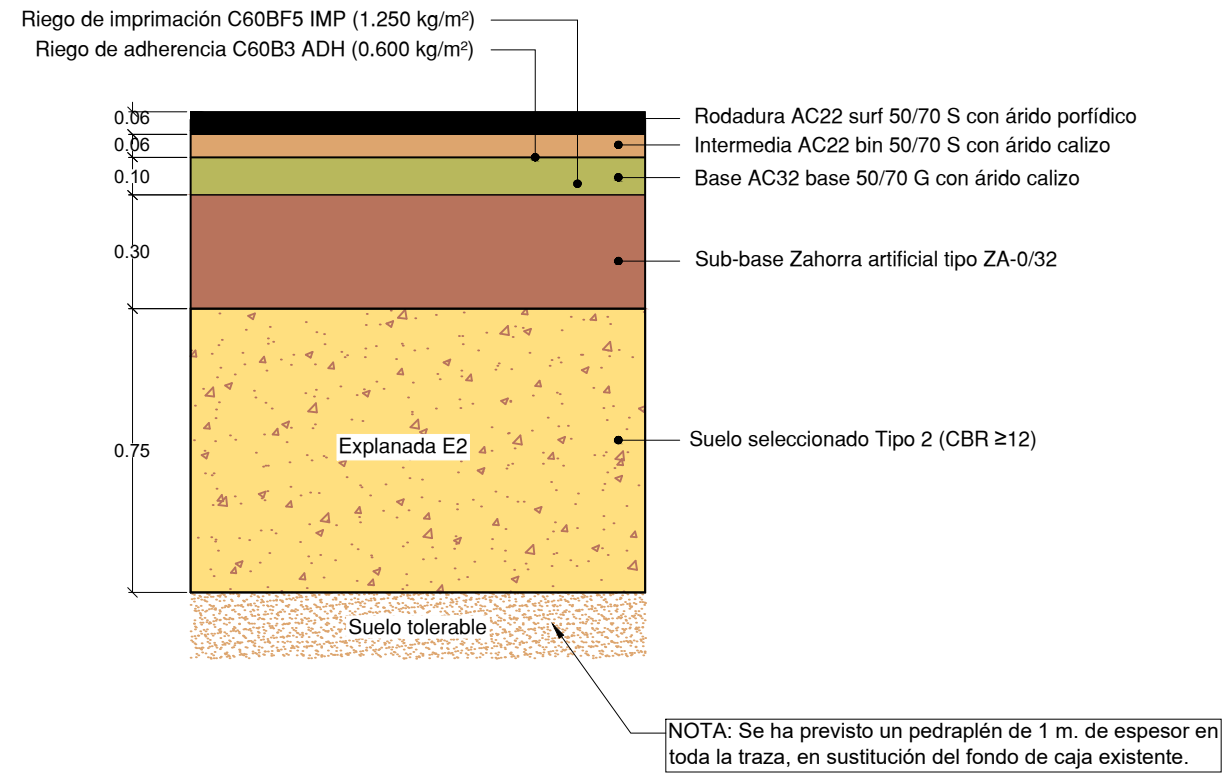
DETALLE 1 – FIRME 2221: Calzada y arcenes \leq 1,00 m.
