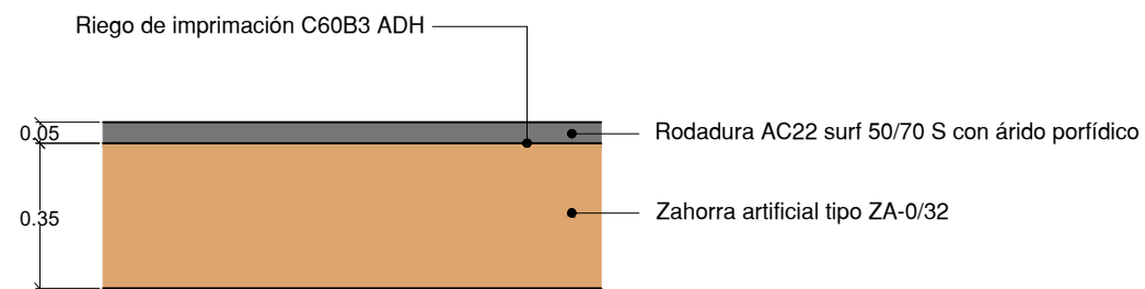
DETALLE 3 - FIRME 4221: Vías ciclo-peatonales
