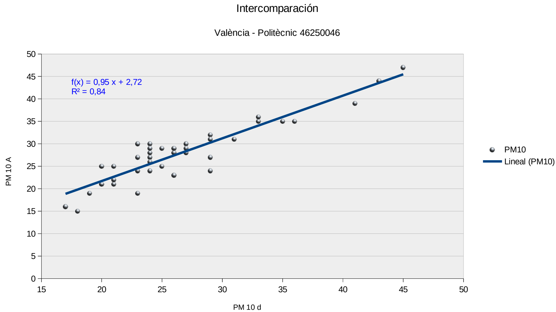
Gràfica 1: Correlació lineal.
