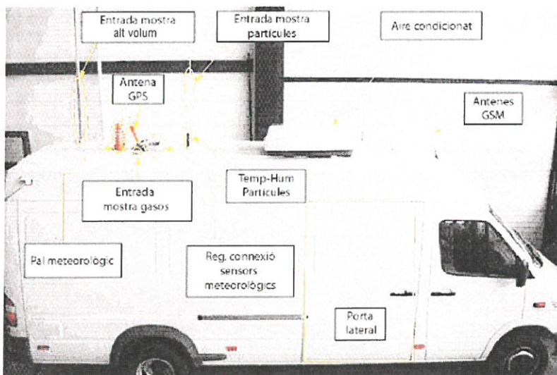
Vista exterior d'una estació mòbil i elements que la formen.
